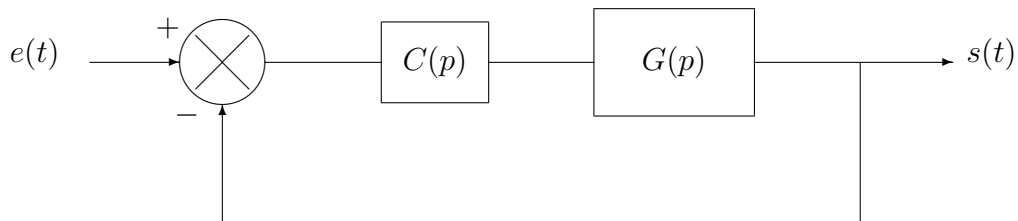
FIGURE 3 – Un système asservi avec correcteur C(p)
