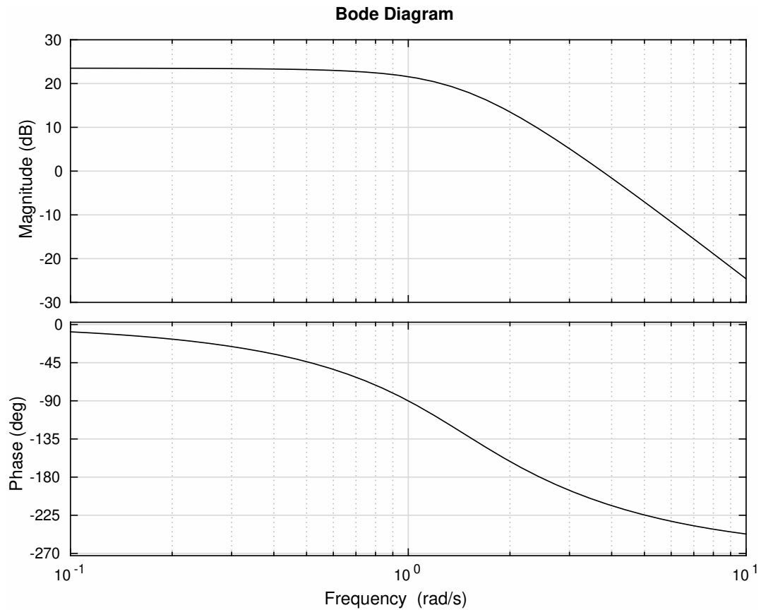
FIGURE 2 – Lieu de Bode de la FTBO tracé pour K = 10 [EXERCICE 1]
