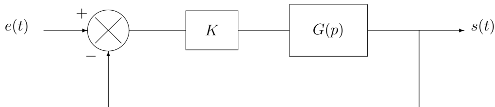
FIGURE 4 – Un système asservi avec correcteur proportionnel
