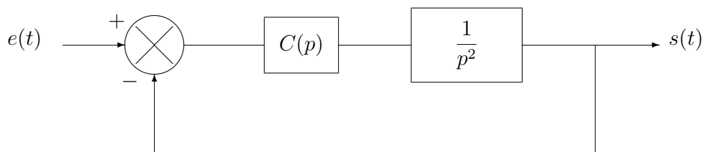
FIGURE 6 – Un système asservi avec correcteur C(p)
