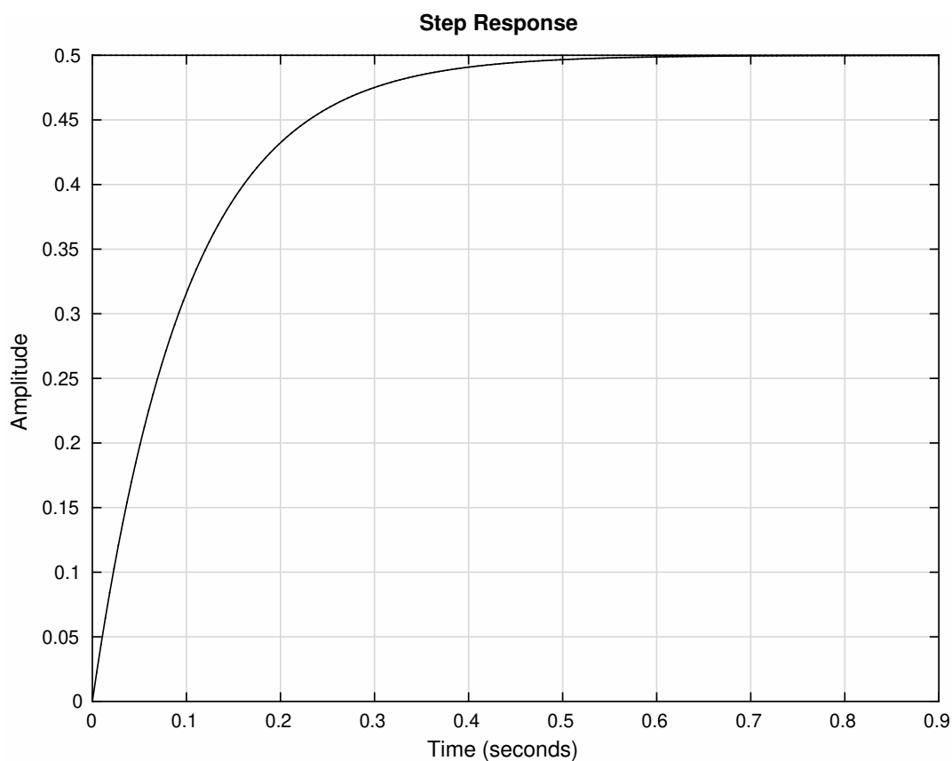
FIGURE 5 – Réponse du système asservi à un échelon unitaire pour K = 2 [EXERCICE 3]
